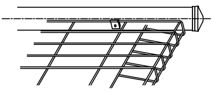
메쉬웬스 상세 조립도
