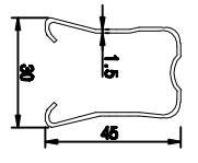
후레이밍 단면 상세도 SCALE : NONE
